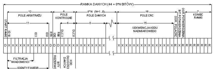
Przykład ramki transmisyjnej CAN
