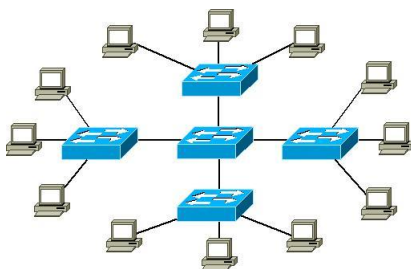
Topologia gwiazdy rozszerzonej
